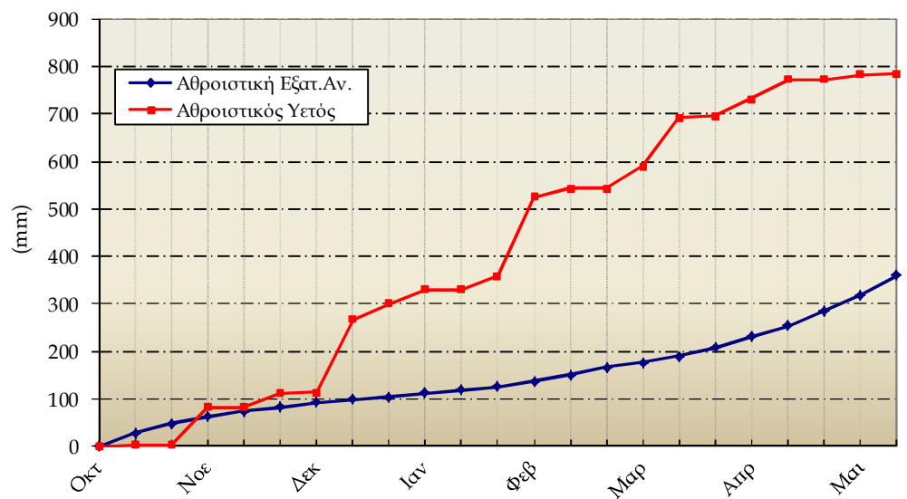
Διάγραμμα Αθροιστικού Υετού και Αθροιστικής Εξατμισοδιαπονης Αναφοράς
